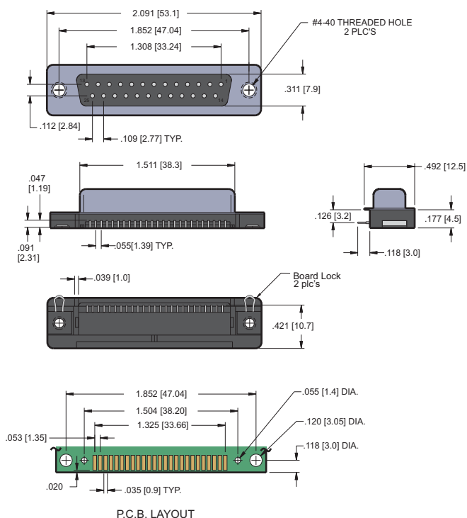
RECEPTACLE
