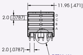
PRESS FIT TAIL
